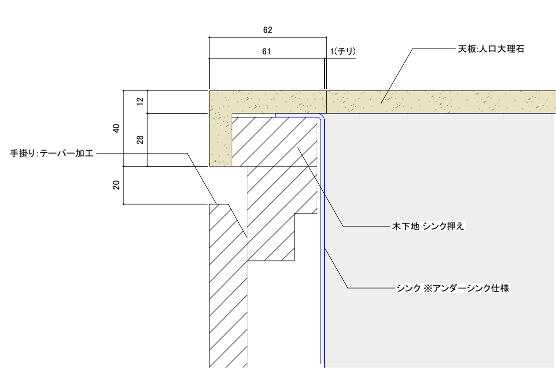
天板断面詳細図
