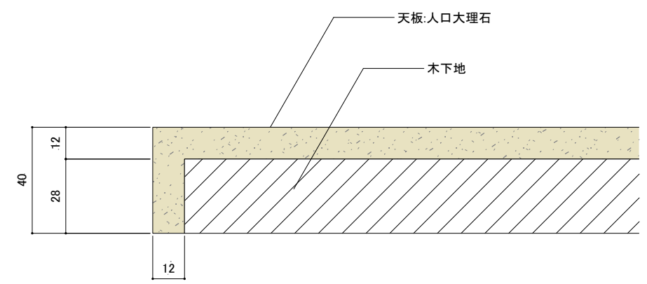
天板断面詳細図
