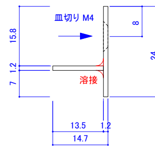
スチール焼き付け塗装 t1.2mm
